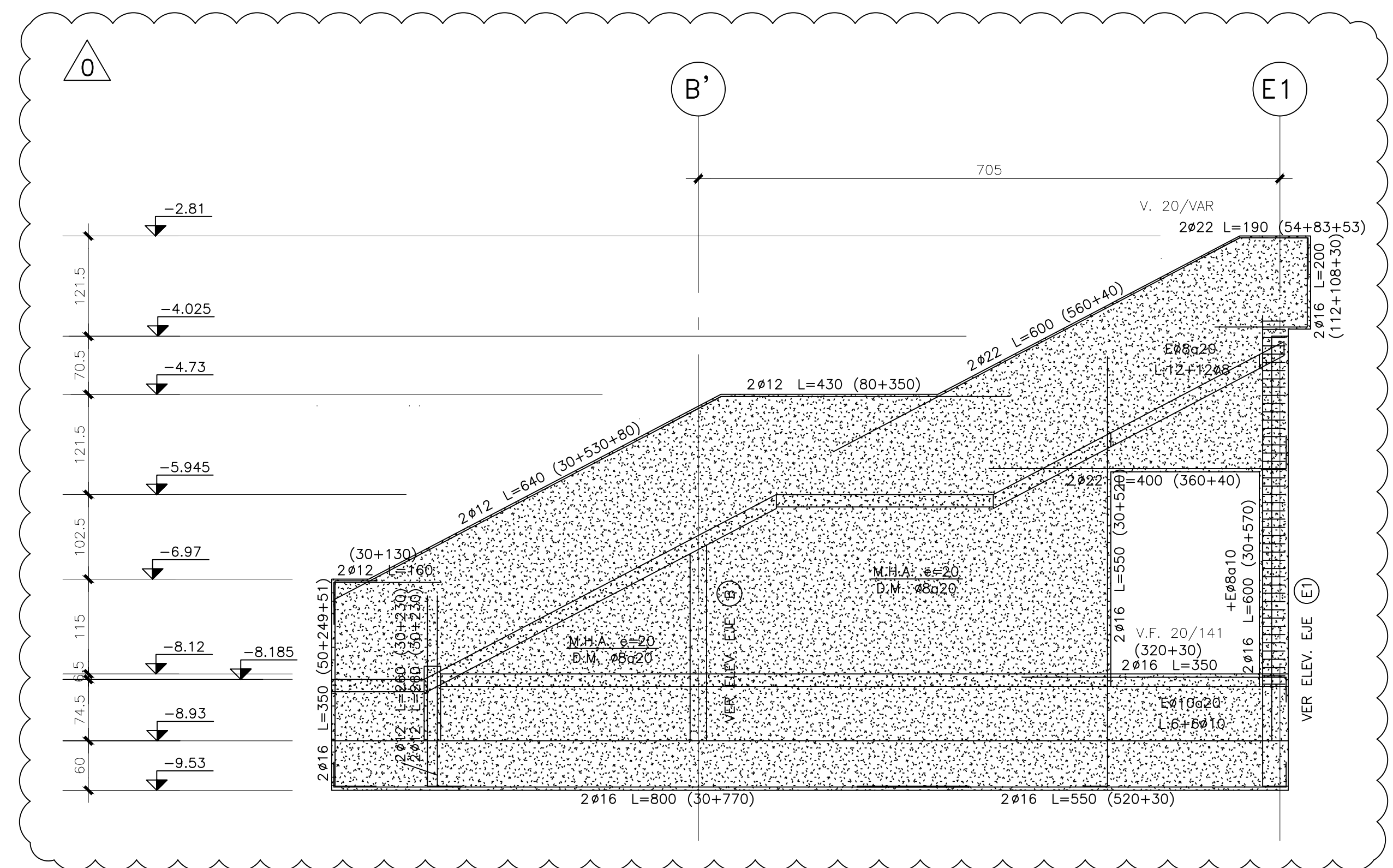
ELEVACION EJE 8A ESCALA 1:50
