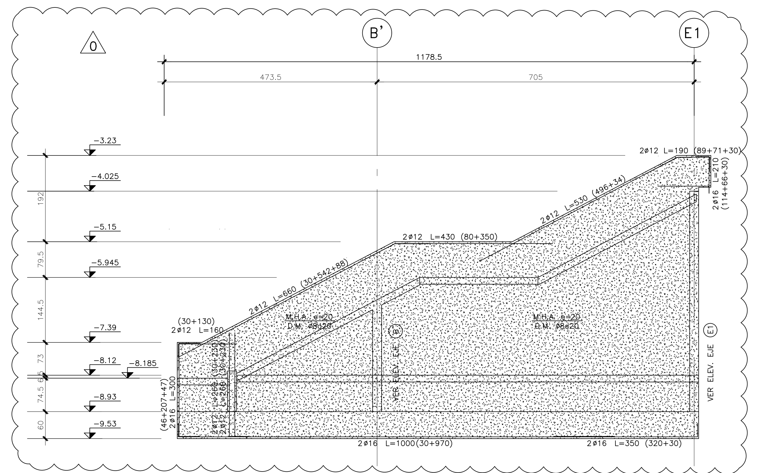
ELEVACION EJE 8B ESCALA 1:50
